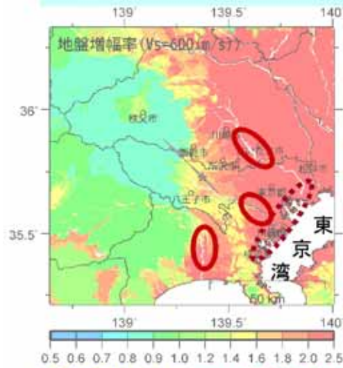
揺れにくい ← → 揺れやすい S波速度 V_s=600\text{ m/s} 相当層に対する表層地盤増幅率分布
