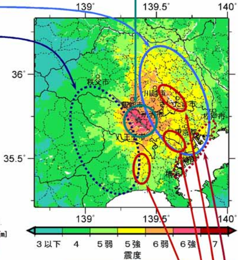
地表面の震度分布
