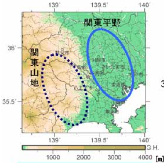
震源断層モデル周辺地形
